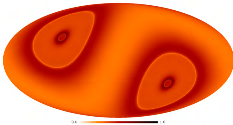
\langle \cos^2(2\beta) \rangle ; polarization w.r.t. NEP; galactic frame
