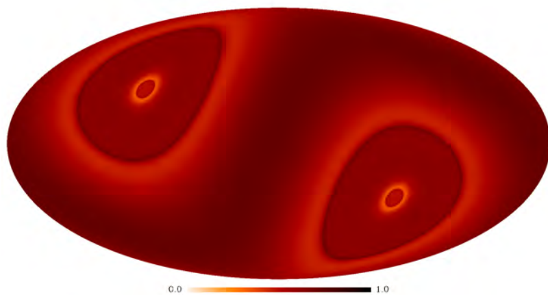
\langle \sin^2(2\beta) \rangle ; polarization w.r.t. NEP; galactic frame
