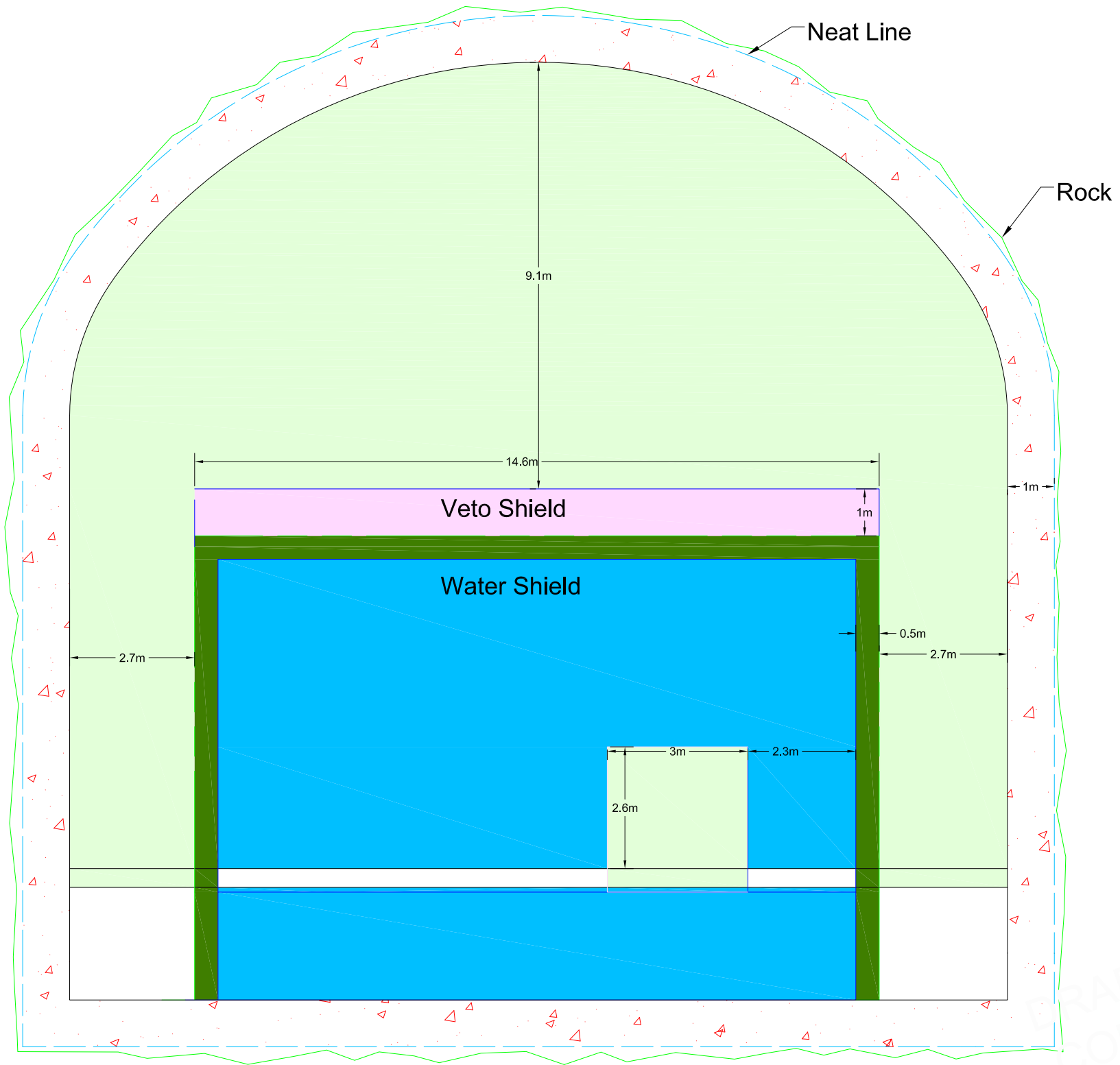
FAARM SECTION BB
